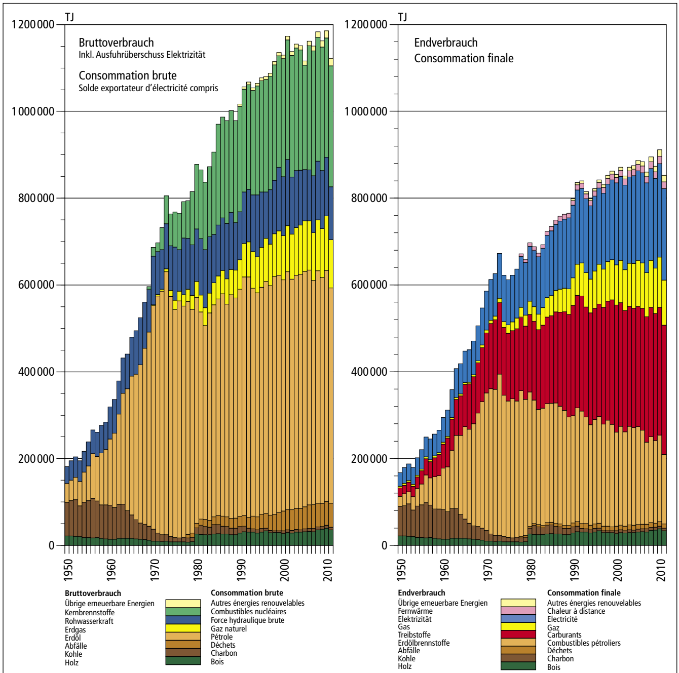
Fig. 4 Energieverbrauch 1950–2011 in TJ Consommation d'énergie 1950–2011 en TJ
