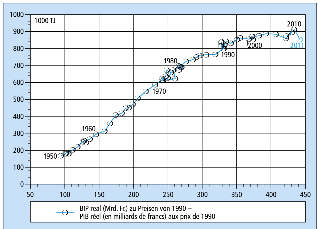
Fig. 15 Zusammenhang zwischen Energieverbrauch und wirtschaftlicher Entwicklung (1950–2011)
