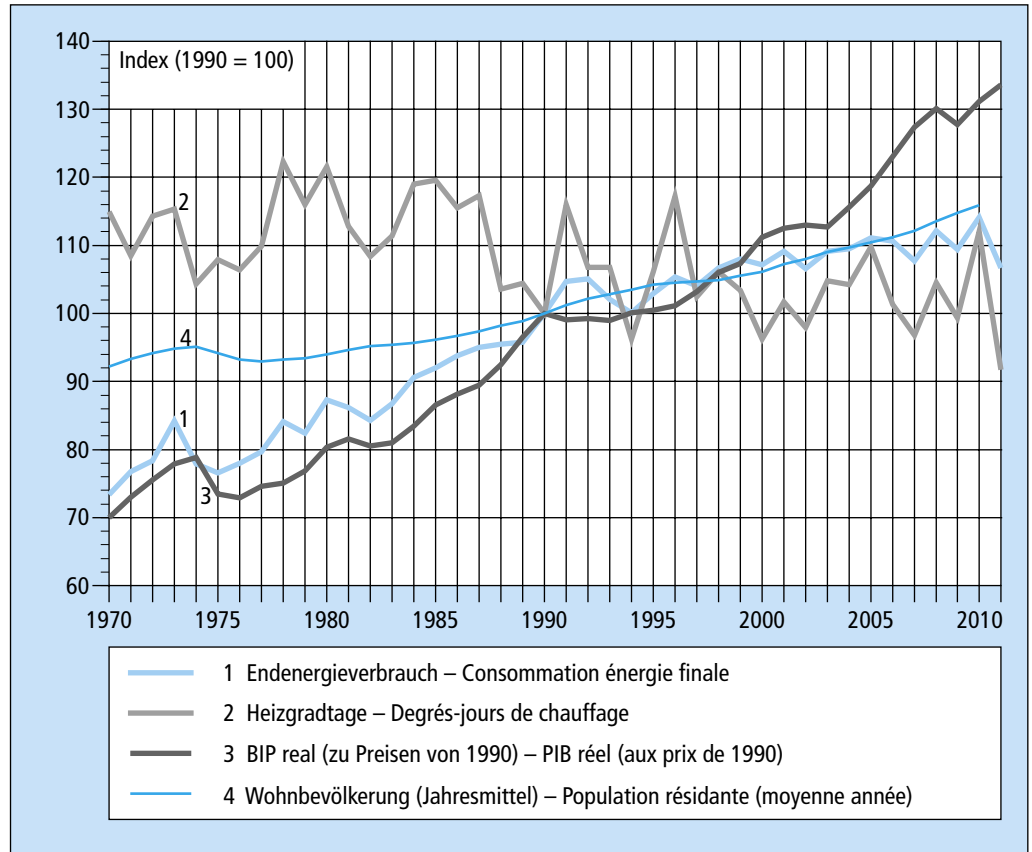
Fig. 14 Entwicklung energierelevanter Größen im Vergleich zum Endverbrauch
